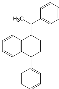
Styrene Trimer
